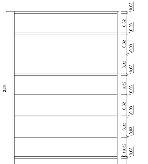
VISTA A- FRONTAL medidas em metros
