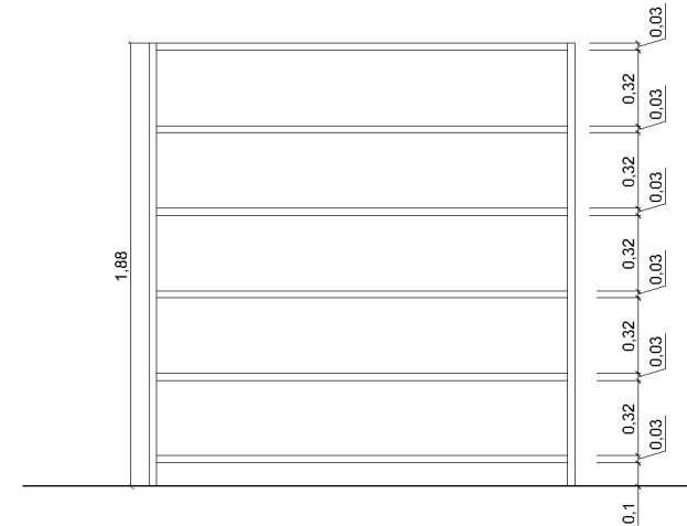
VISTA B - FRONTAL Medidas em metros
