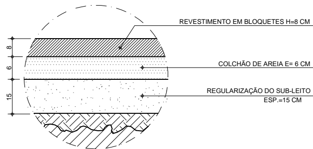
DETALHE 1- CORTE CAMADAS – BLOQUETE sem escala
