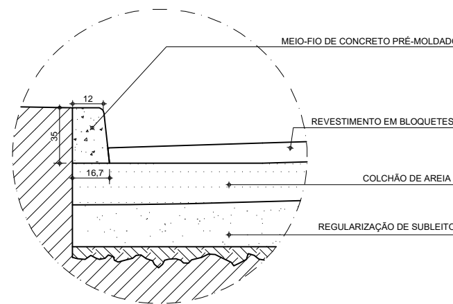
DETALHE 2- MEIO FIO E BLOQUETE sem escala
