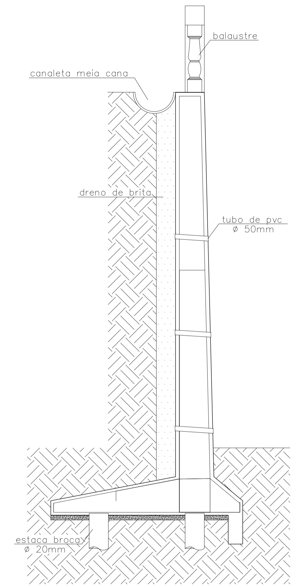
DETALHE GENÉRICO escala 1/50
