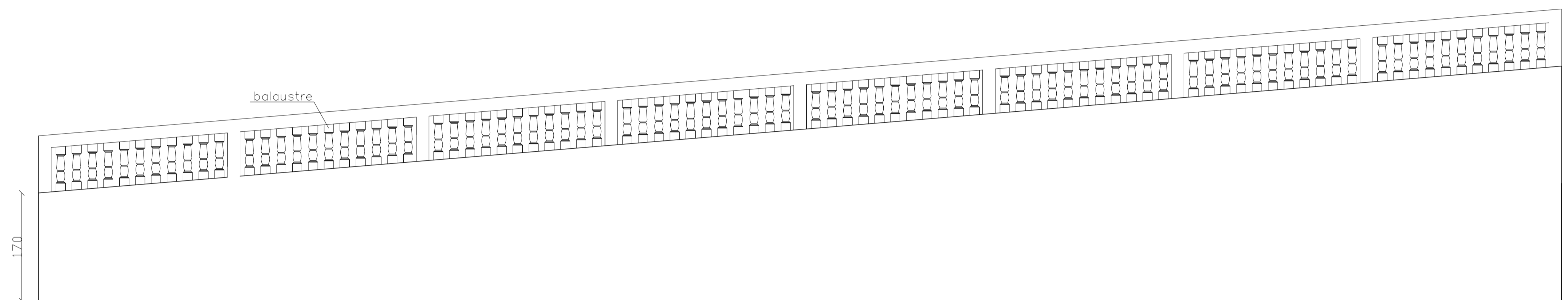
FACHADA DO MURO escala 1/100
