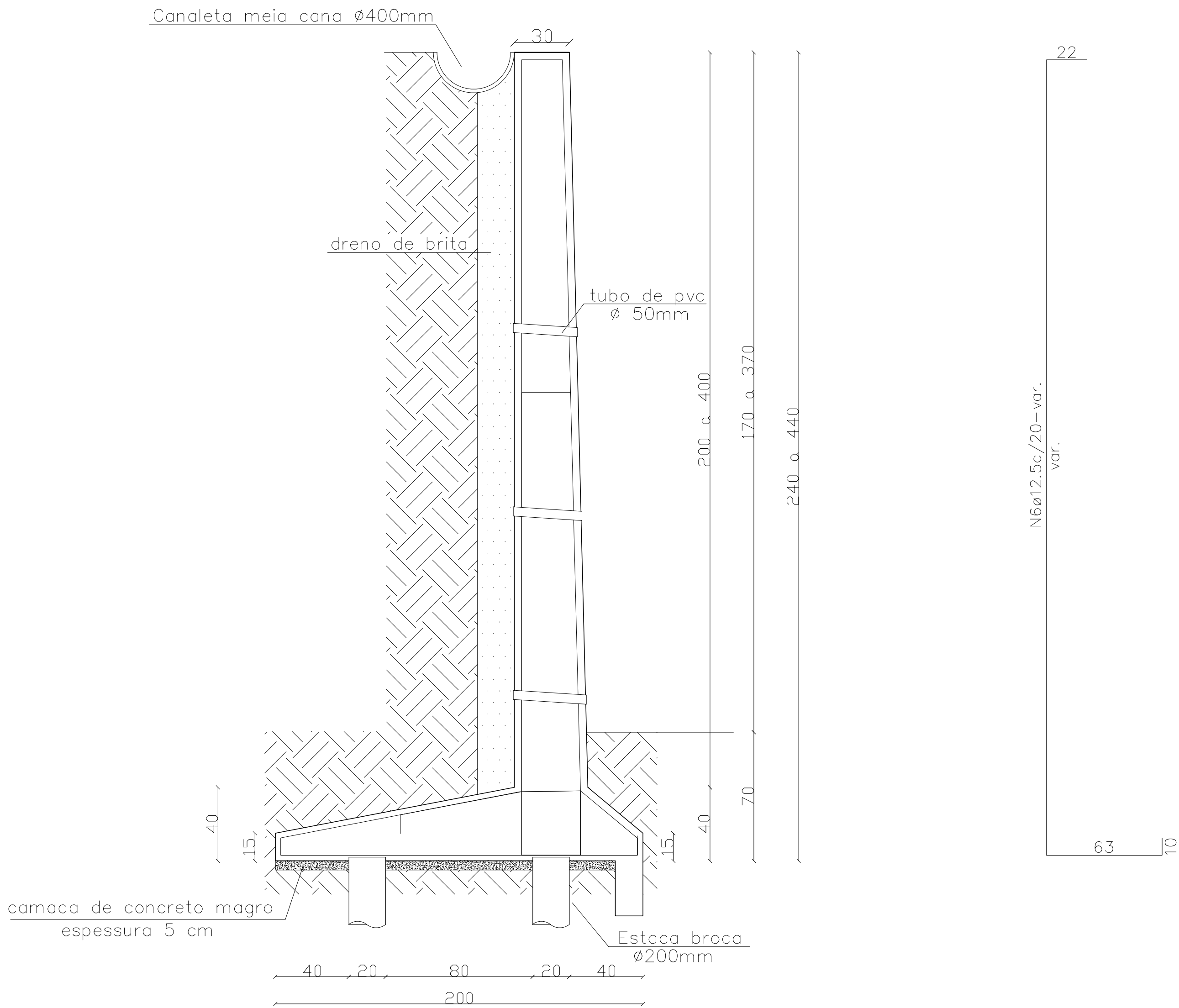
PLANTA DE FORMA escala 1/50
