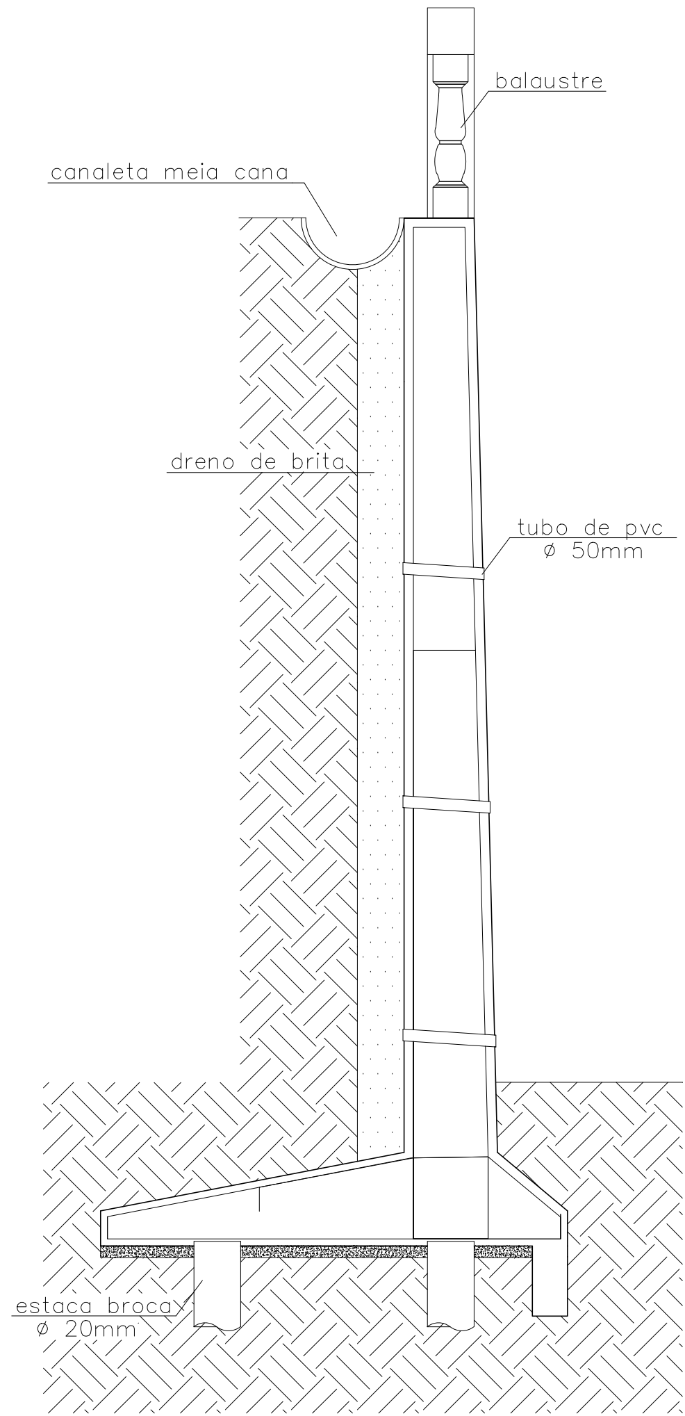
DETALHE GENÉRICO escala 1/50
