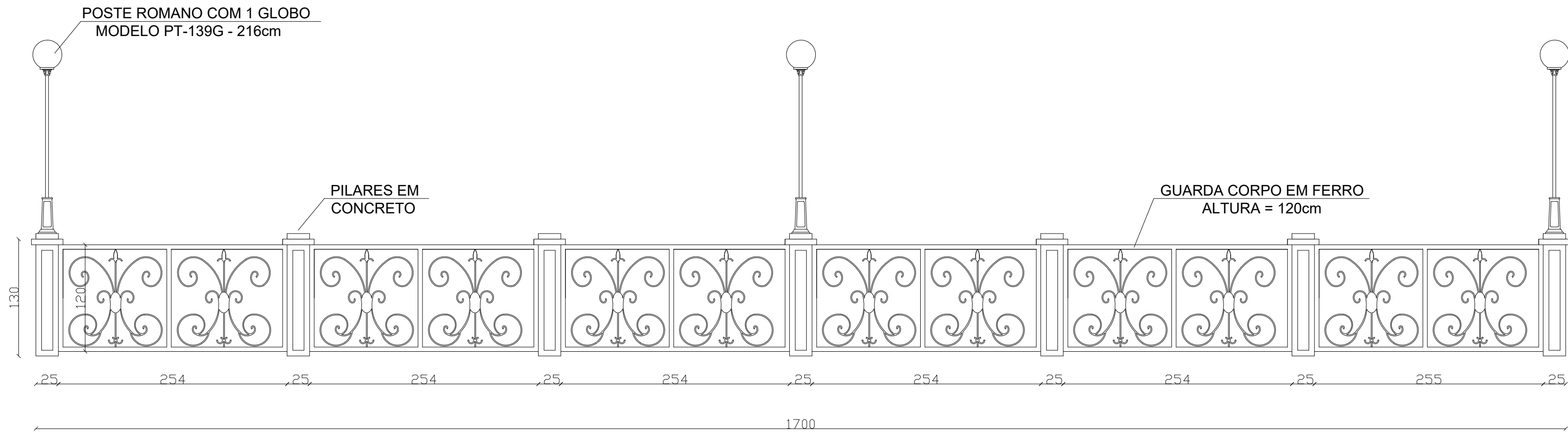
DETALHE GUARDA CORPO DA PONTE - MODELO 01 sem escala
