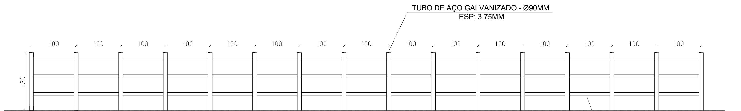
DETALHE GUARDA CORPO - MODELO 02 sem escala
